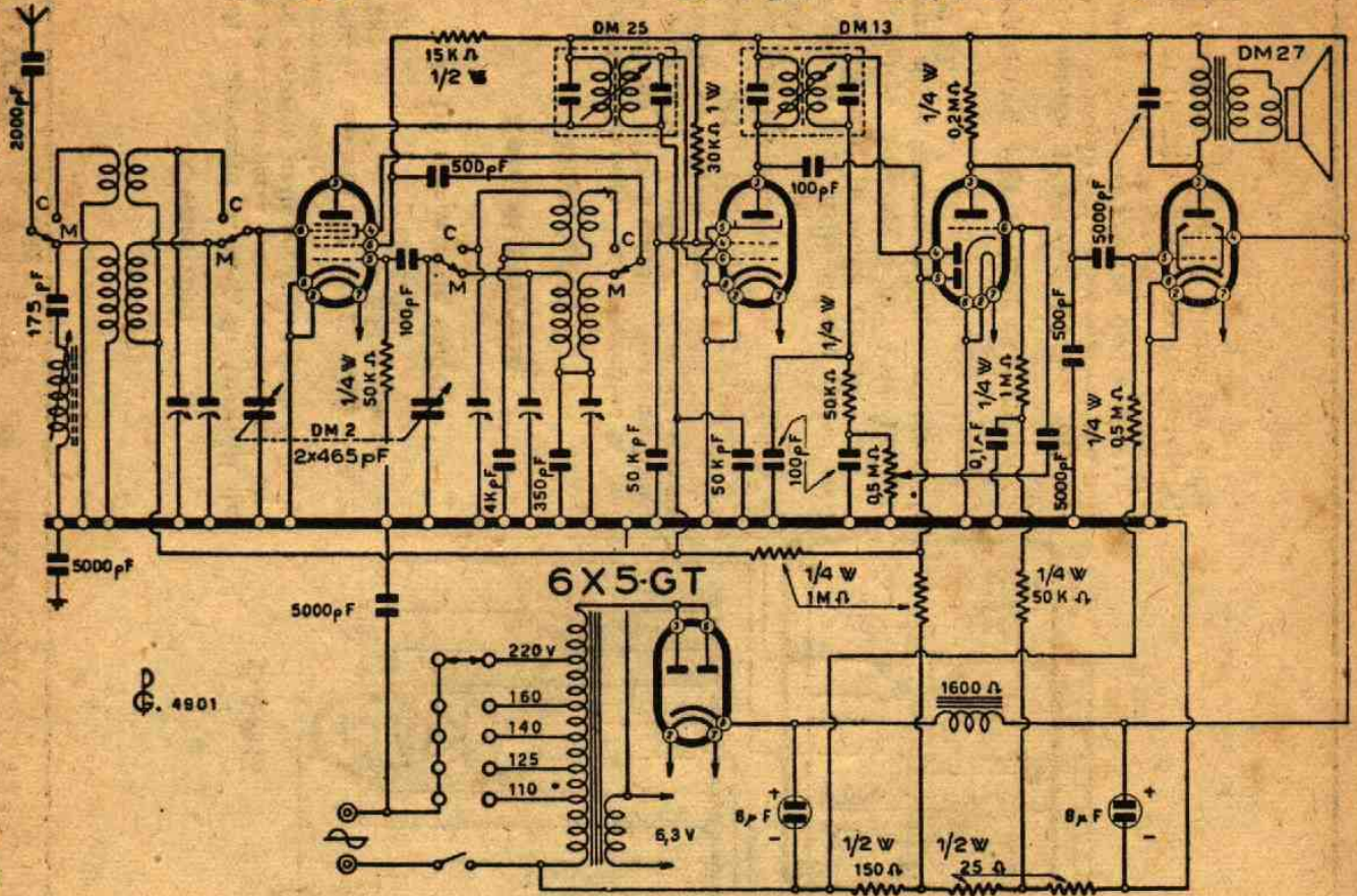
Lo schema del mod. "523 Milly"
