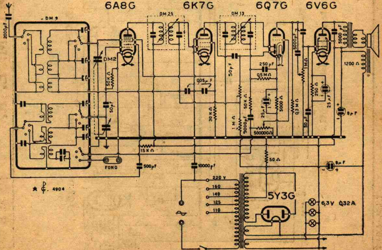
Lo schema del mod. "532"
